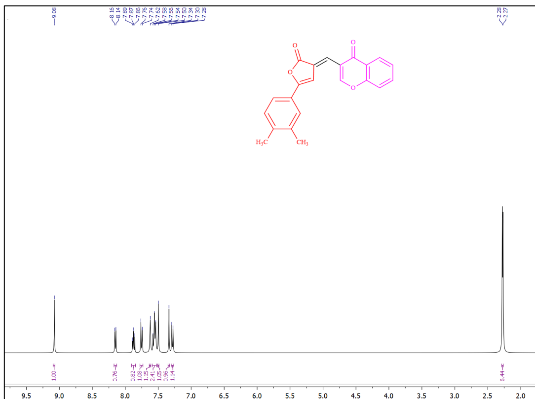
Fig. S5. ^1\text{H} & ^{13}\text{C} of 3e
