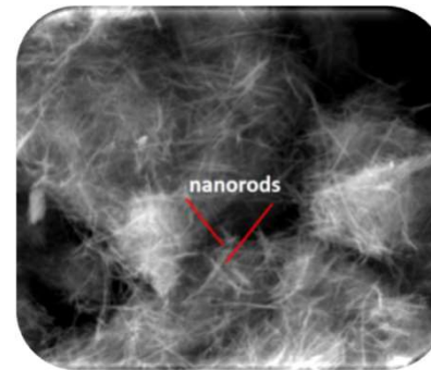
Urchin-MnO 2
