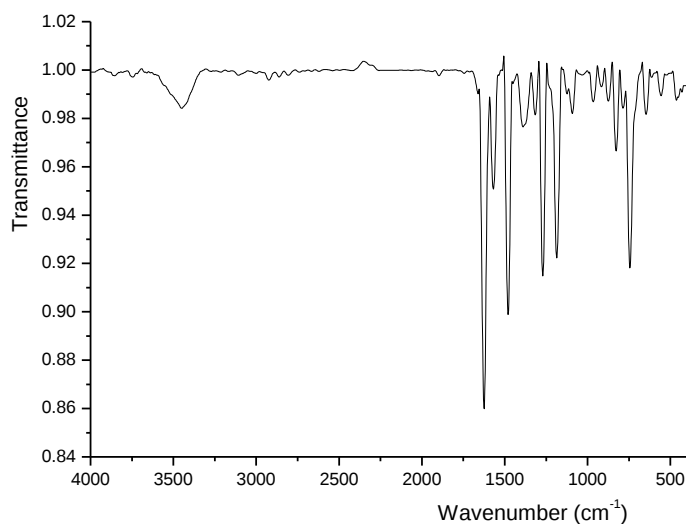
Fig. S1. IR spectrum of H 2 L.
