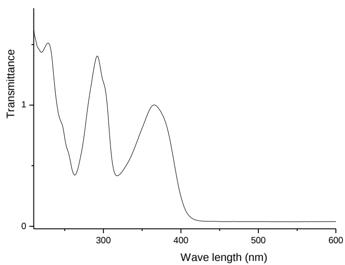
Fig. S4. UV-Vis spectrum of H 2 L.
