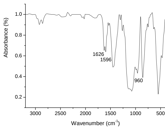
Fig. 3. IR spectrum of complex 2.
