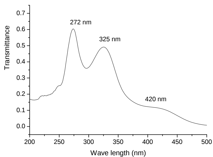
Fig. 4. UV-Vis spectrum of H 2 L.
