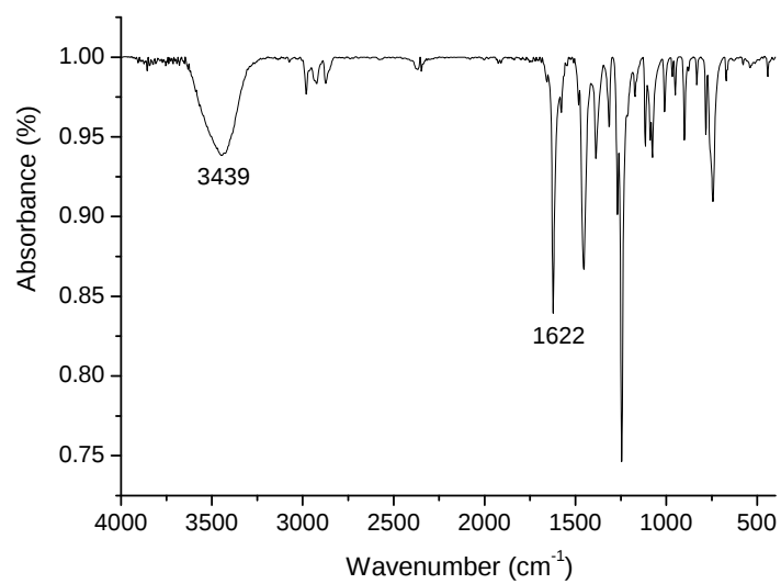
Fig. 1. IR spectrum of H_2L .
